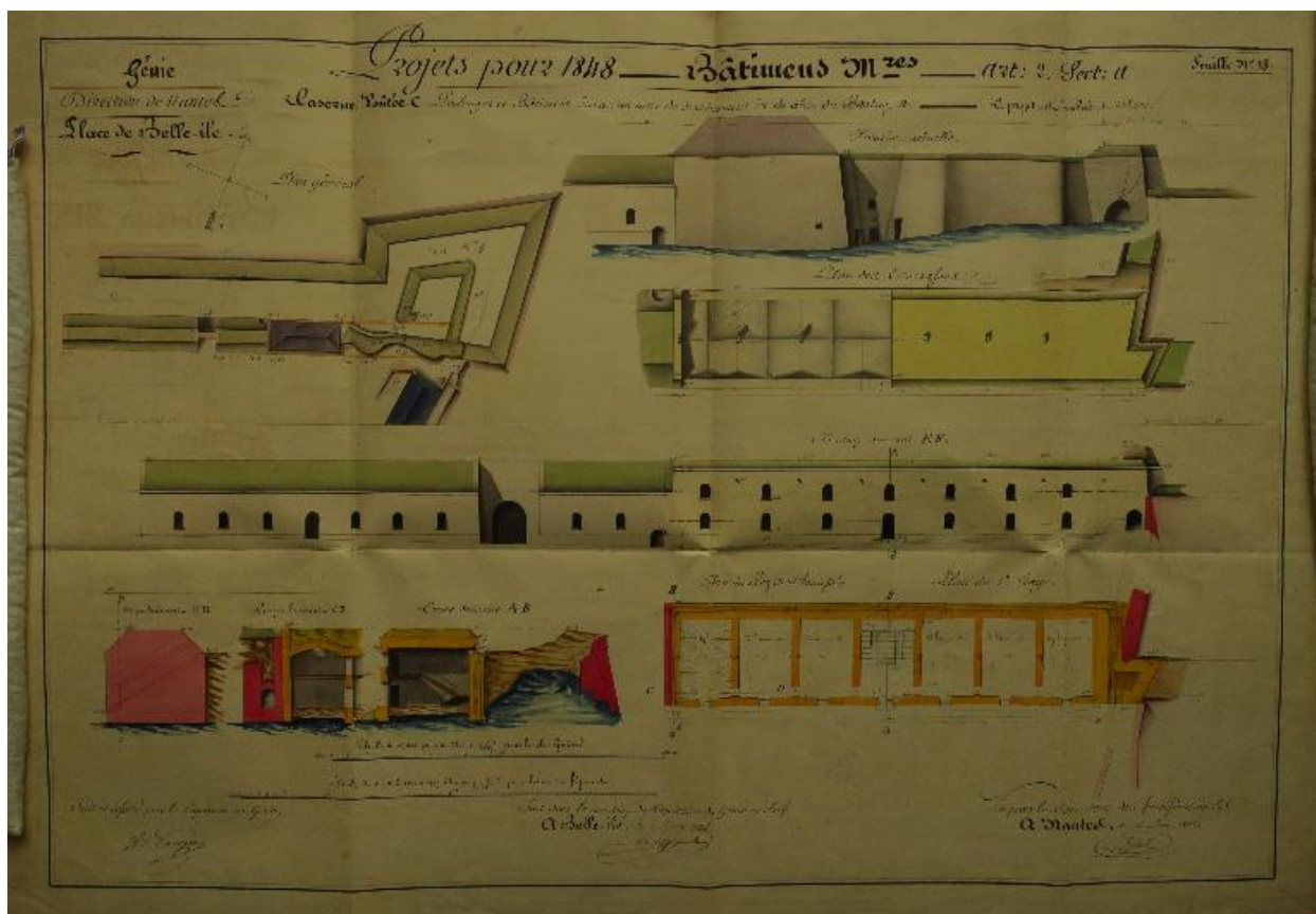
Place de Belle-Ile, feuille n° 18 des projets pour 1848, prolongement de la caserne voûtée C, 5 juin 1848.
