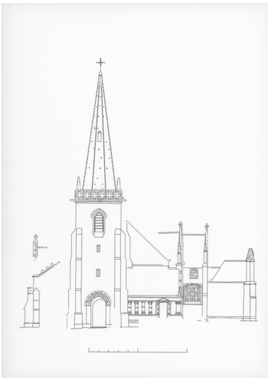
Elévation de la façade occidentale, photogrammétrique
