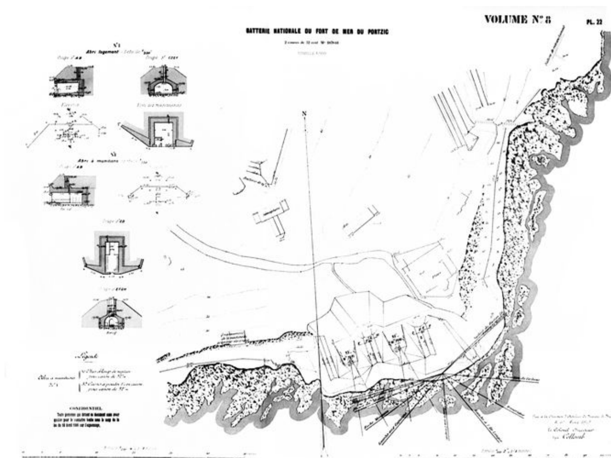
Plan et coupes de la batterie Nationale du fort de mer du Portzic (2 canons M de 32 cm modèle 1870-1881), Direction d'Artillerie du génie de Brest, 1893, par le colonel Directeur d'Artillerie : Collomb
