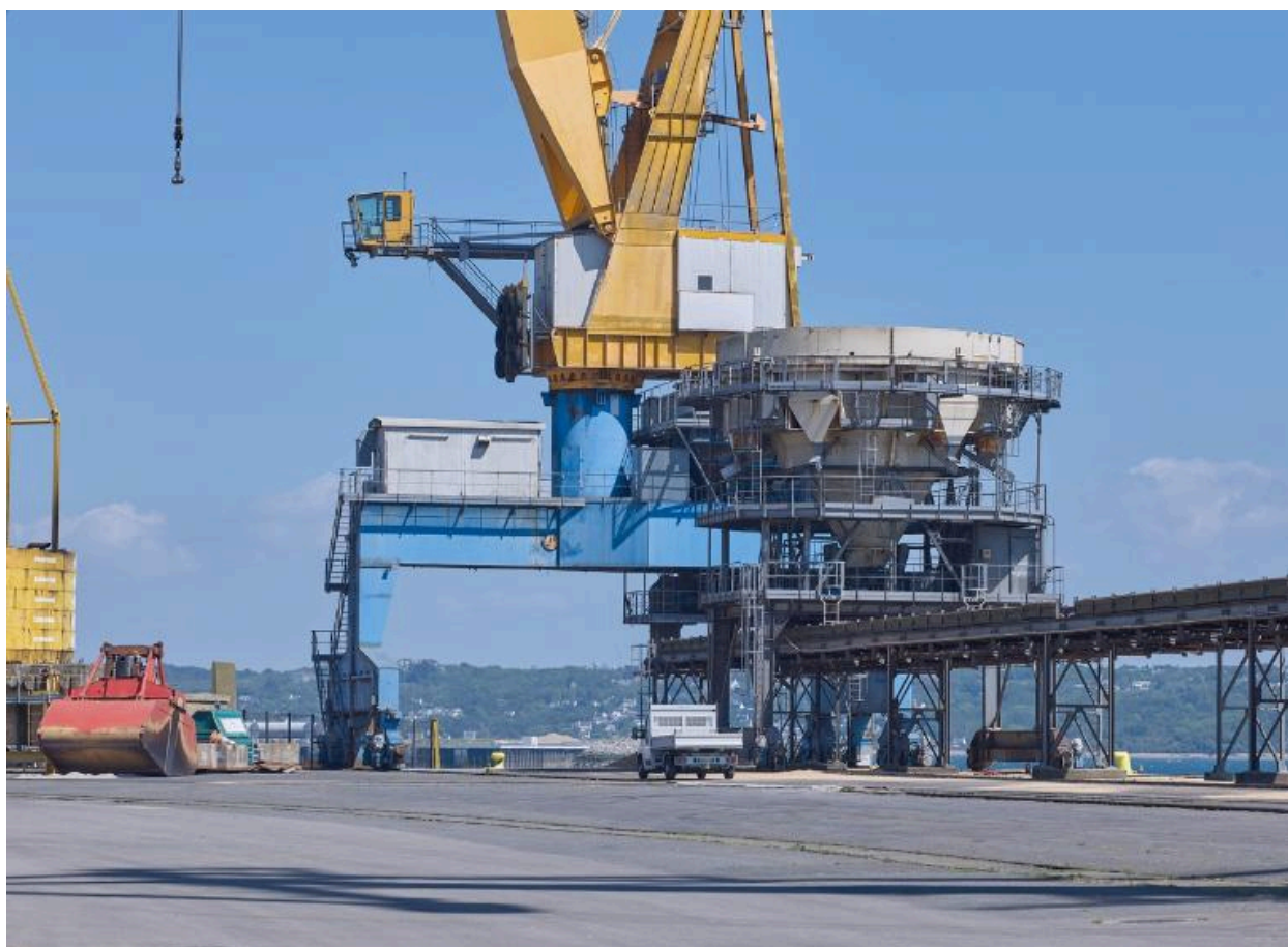
Trémies et grues quai 6e sud
