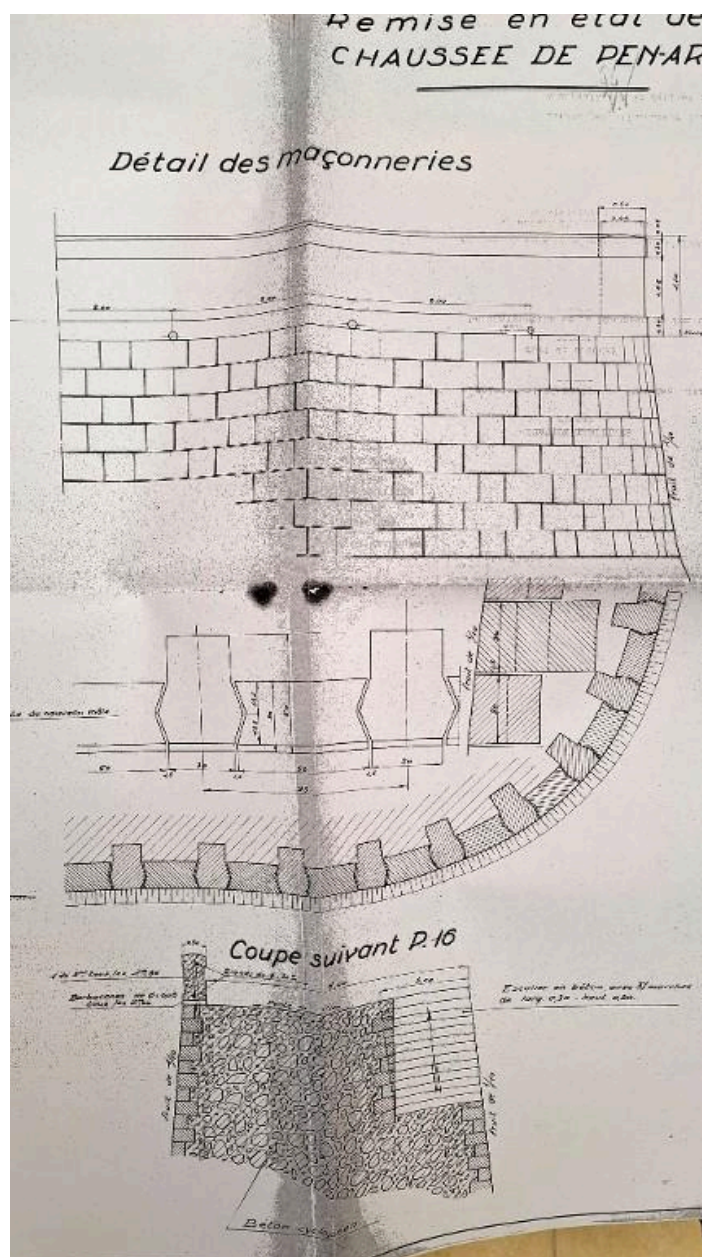
Profil en long de l'extrémité de l'ouvrage de Pen ar Vil : détail des maçonneries, juillet 1947
