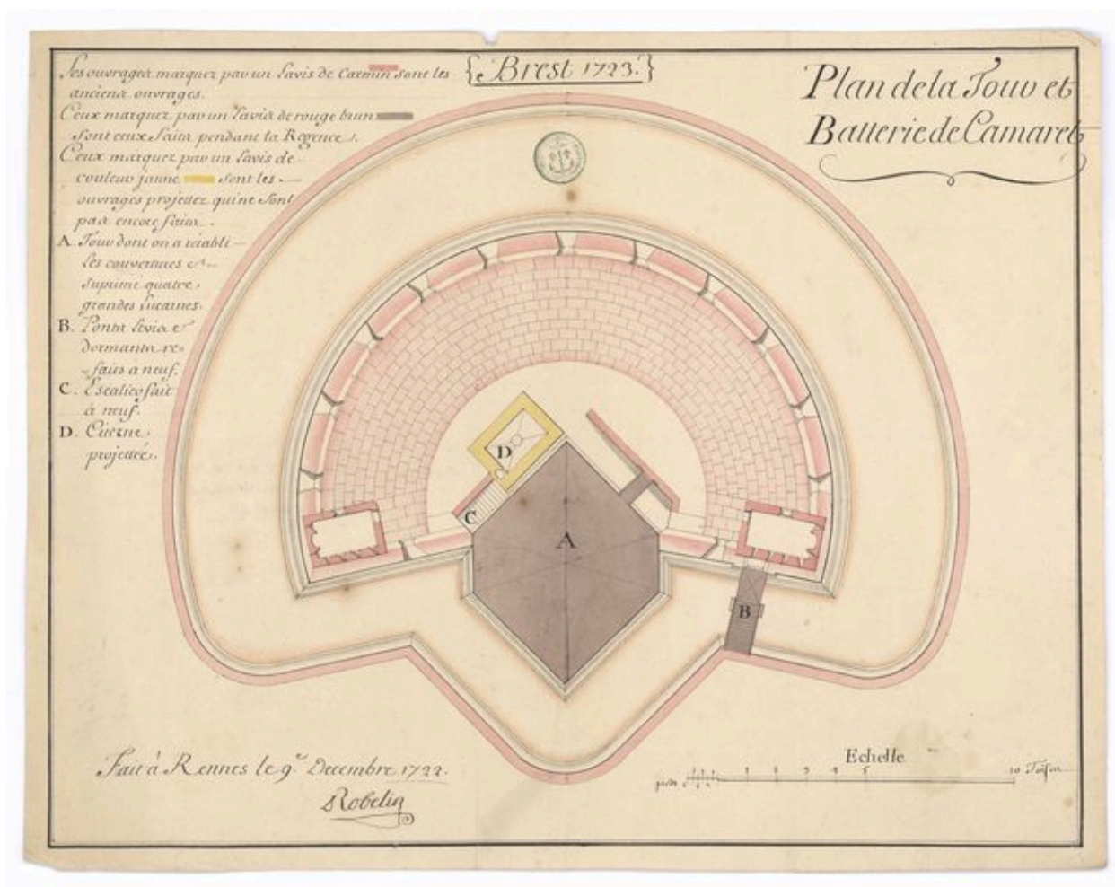
Plan de la tour et de la batterie de Camaret, projet de citerne, fait à Rennes le 9 décembre 1722 par Robelin
