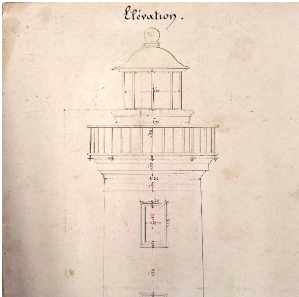
Plan : élévation du phare de la pointe de l'Aigle, 29 novembre 1851 (extrait)
