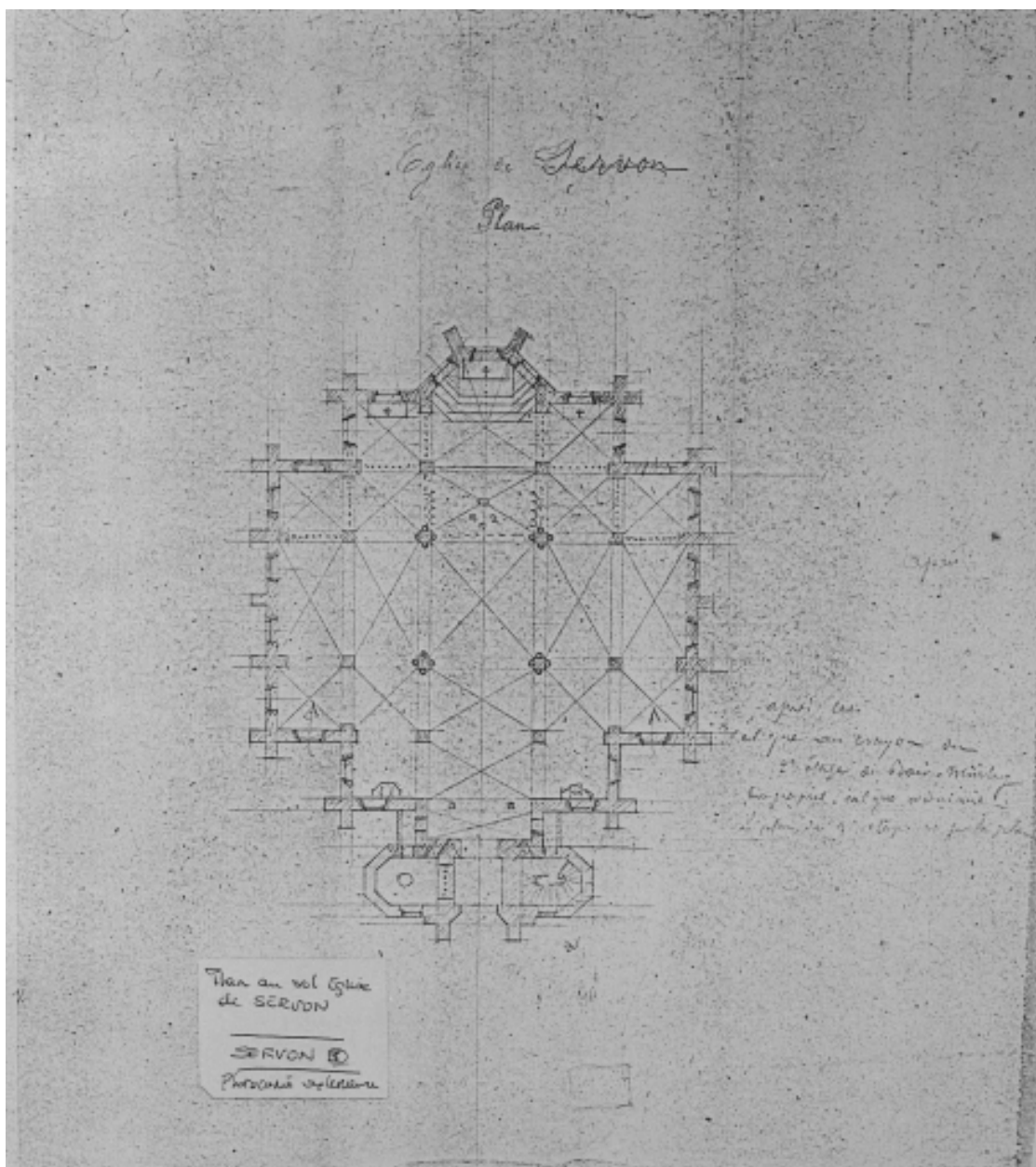
Plan au sol, attribué à A. Regnault
