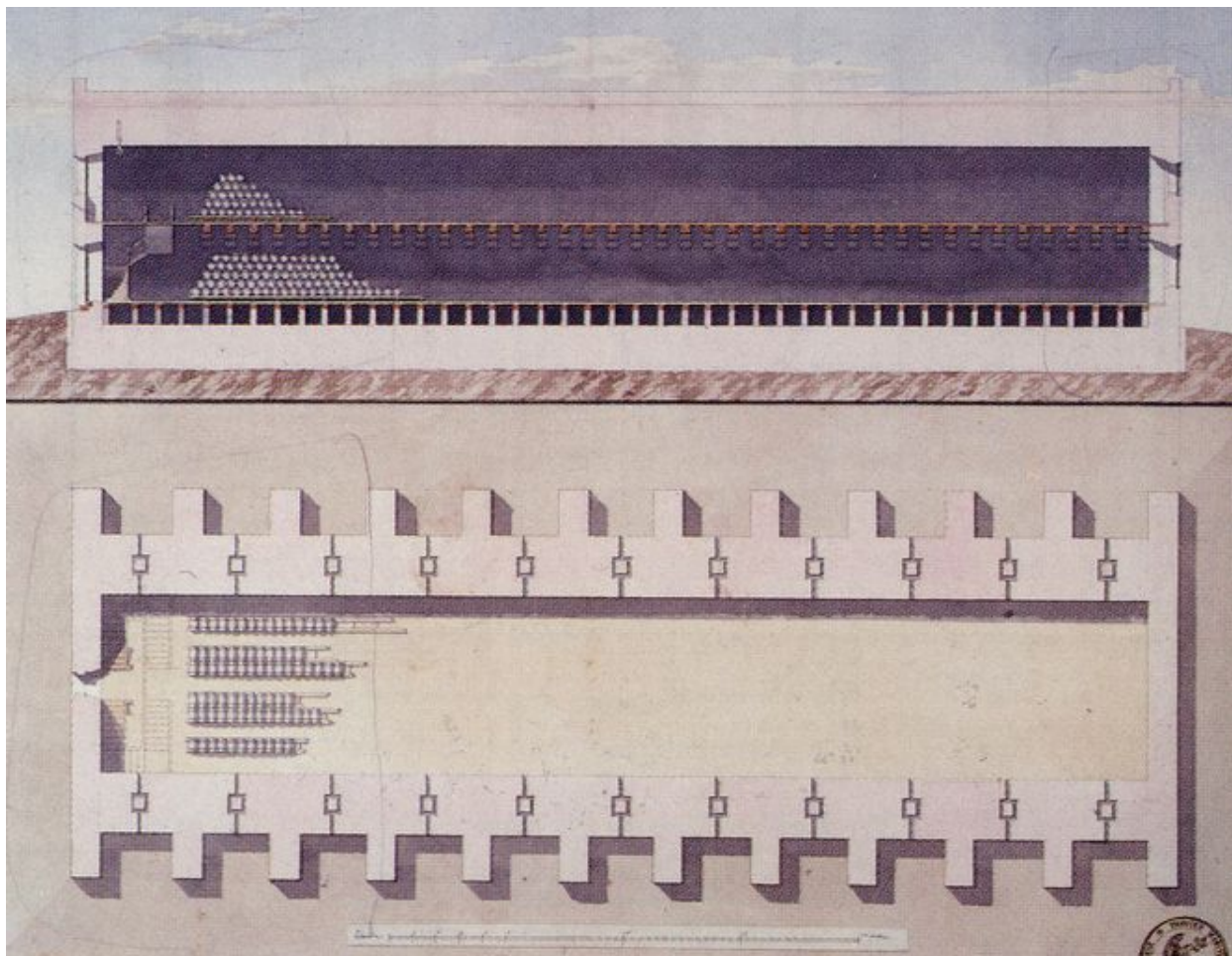
Plan et coupe de l'un des trois magasins à poudre dits "poudrières maritimes" de l'île des Morts, Travaux Maritimes, 1813
