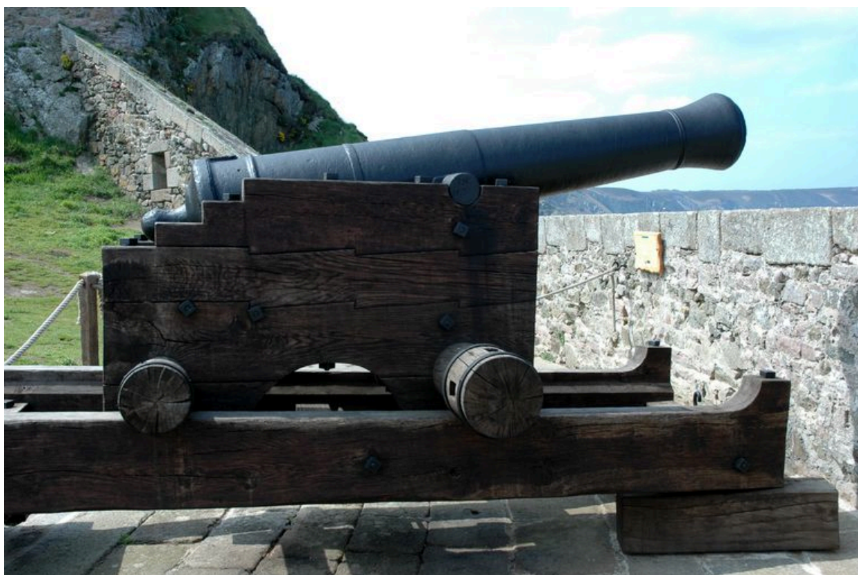
Vue du Fort La Latte : reconstitution d'un canon sur affût à châssis pivotant type Gribeauval
