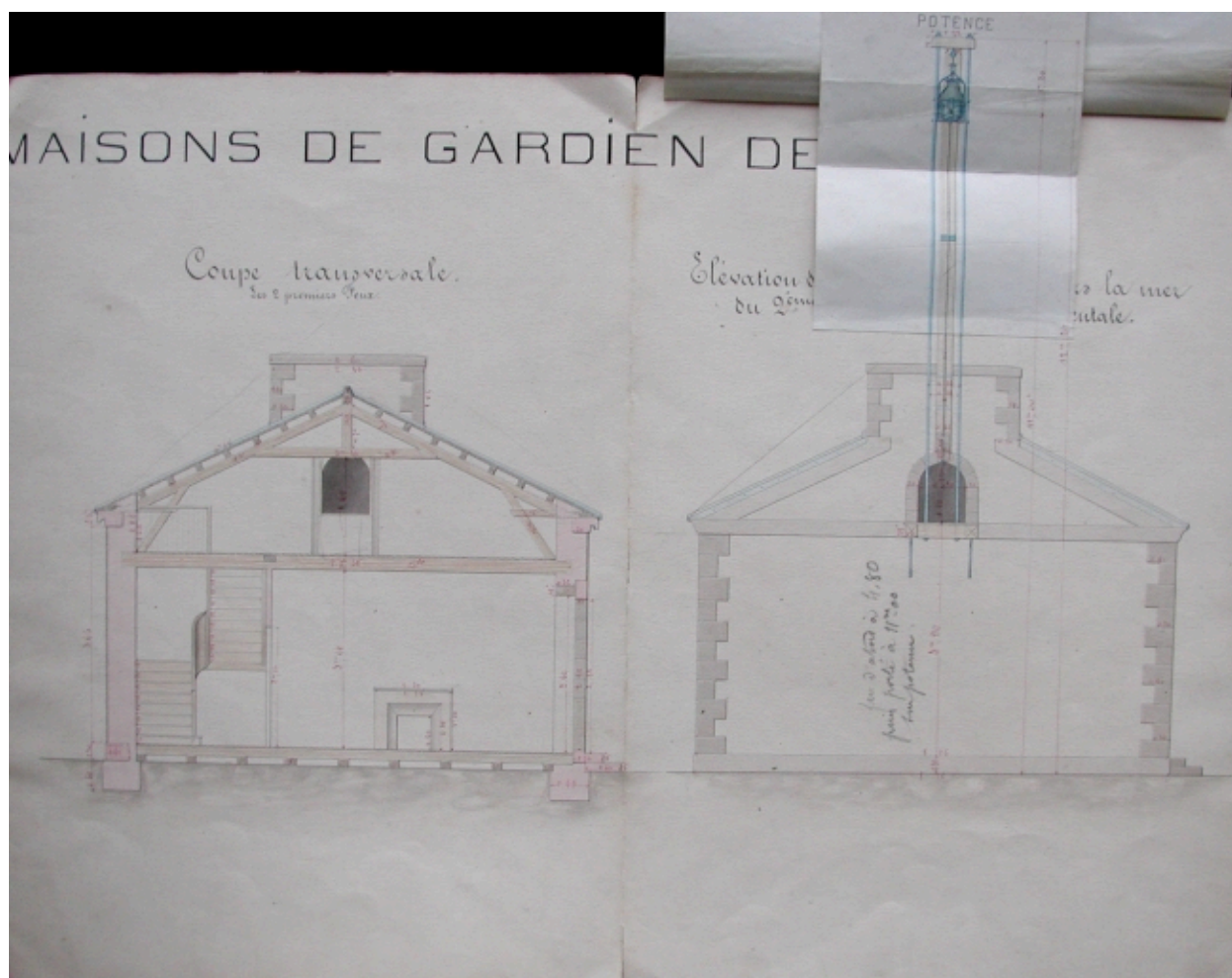
Elévation et coupe transversale de la maison-phare, 1857 : remarquer la potence (AD 22)
