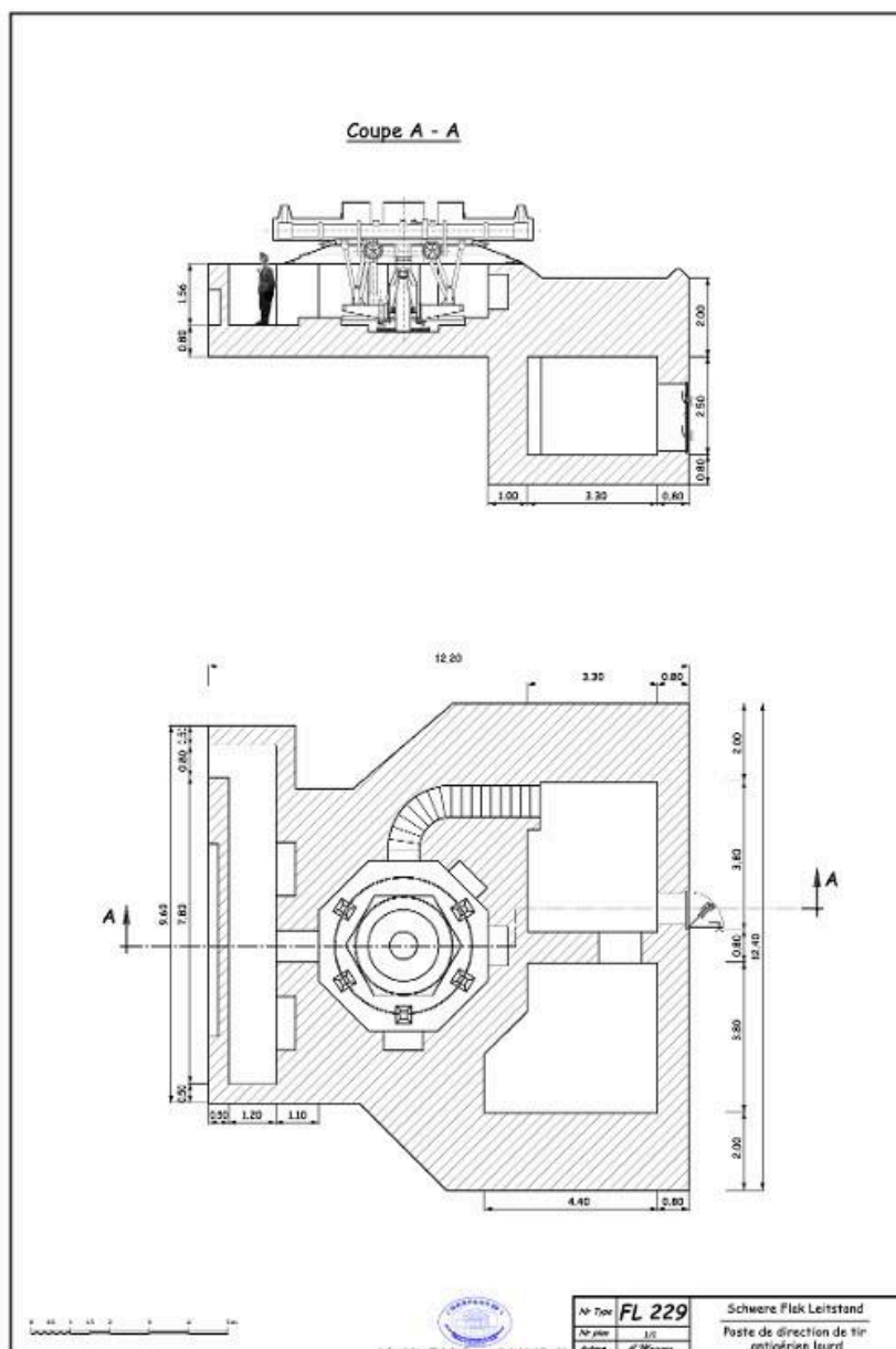
Plan et coupe d'un bunker-poste de direction de tir de type FI 229 pour batterie antiaérienne lourde (Schwere Flak Leitstand)
