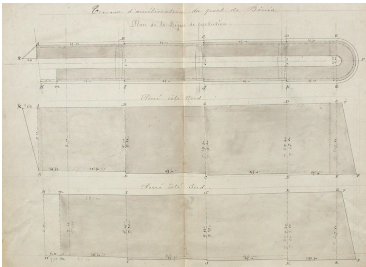
Plan et profils des perrés de la digue de protection (AD 22)
