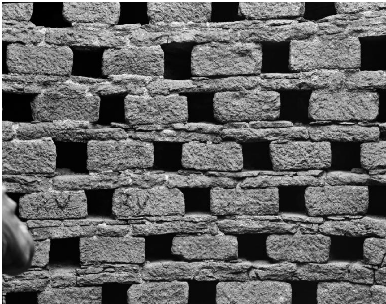
Colombier, détail trous de boulins
