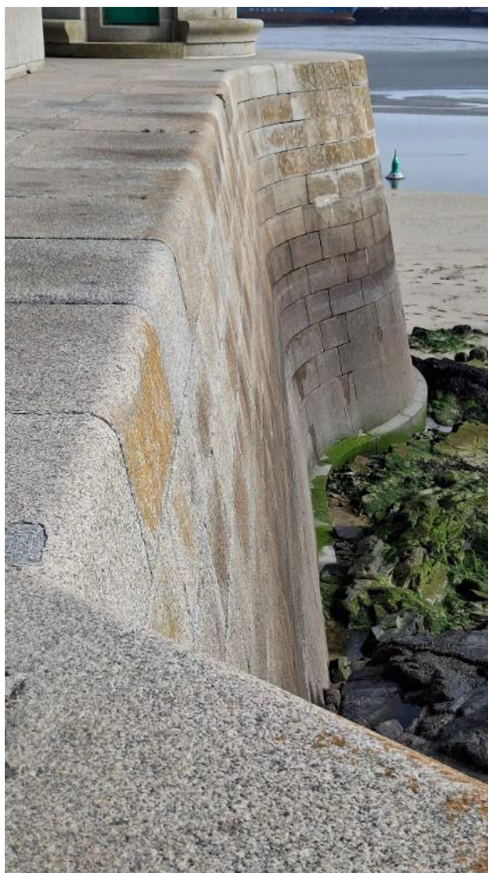
Détails des maçonneries de la jetée
