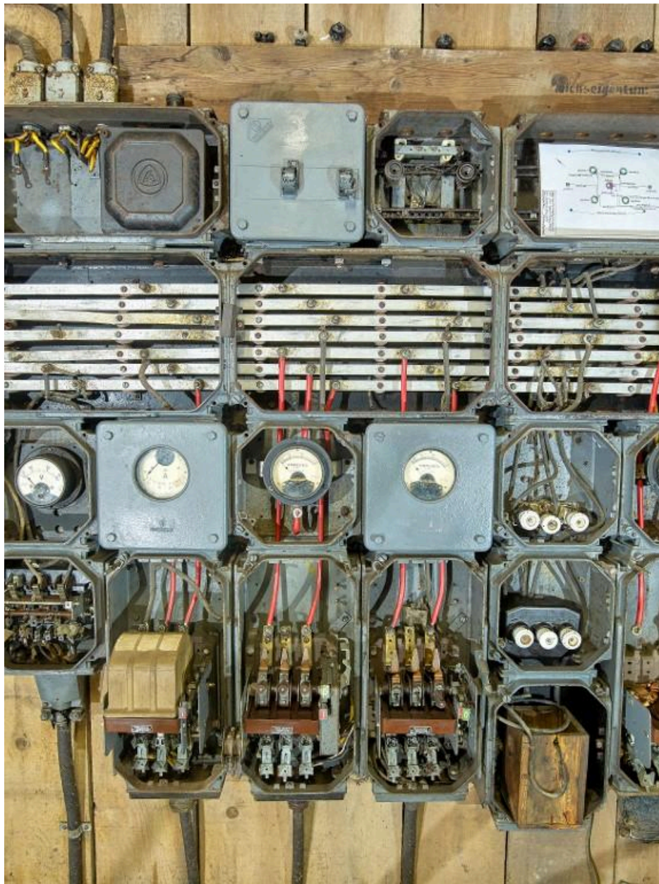
Vue intérieure : salle des machines pour deux groupes électrogènes, détail du tableau électrique de la batterie antiaérienne Rossitten
