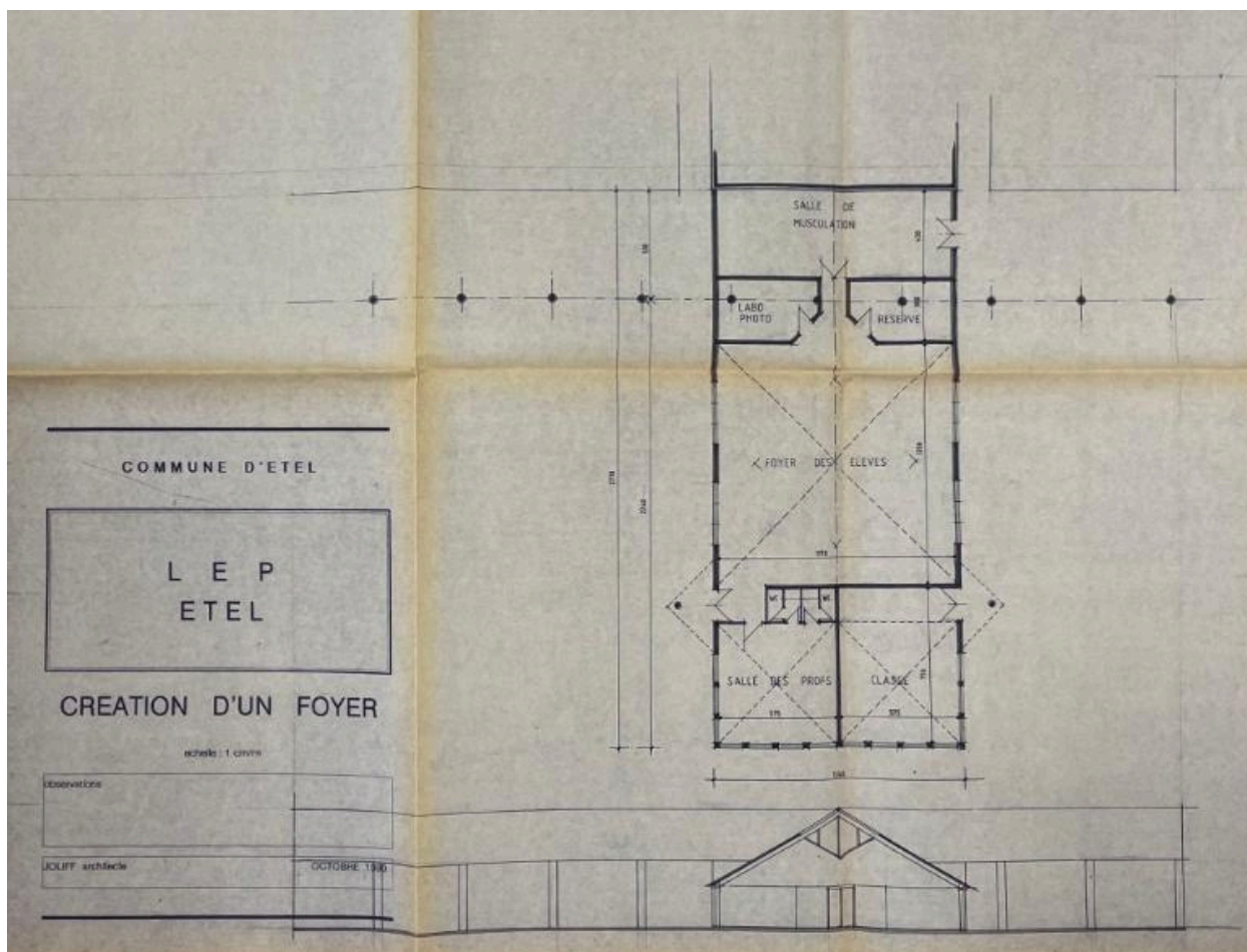
Plan et coupe du foyer des élèves (APS), Christian Joliff, architecte, 1990.
