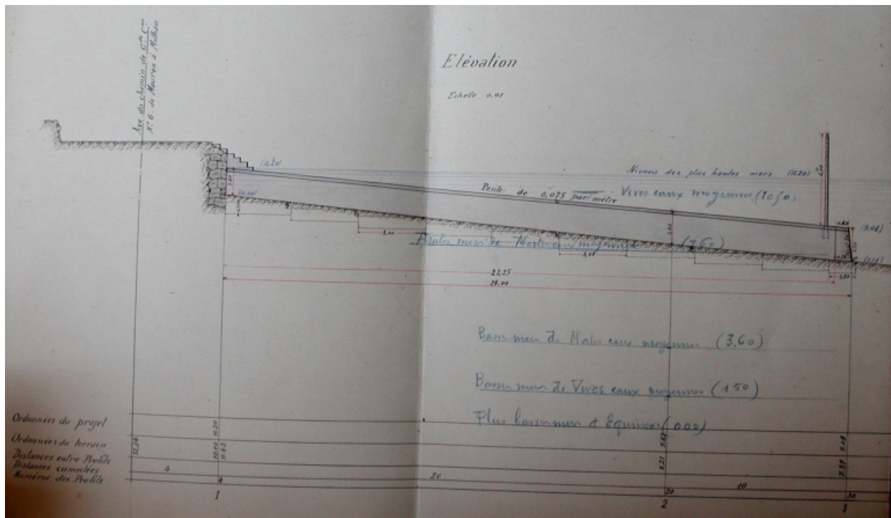
Plan : élévation de la cale projetée, 1912 (AD 22)
