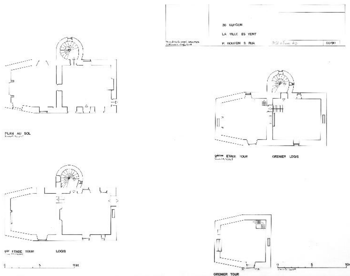
Plans au sol des quatre niveaux (état en 1991)
