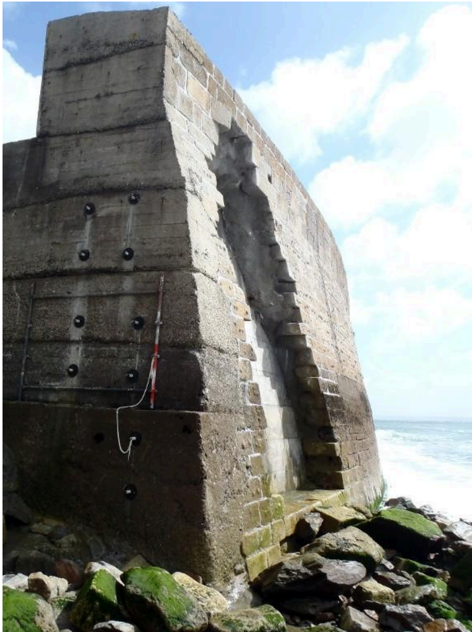
Vue de la brèche après les travaux de consolidation de 2015
