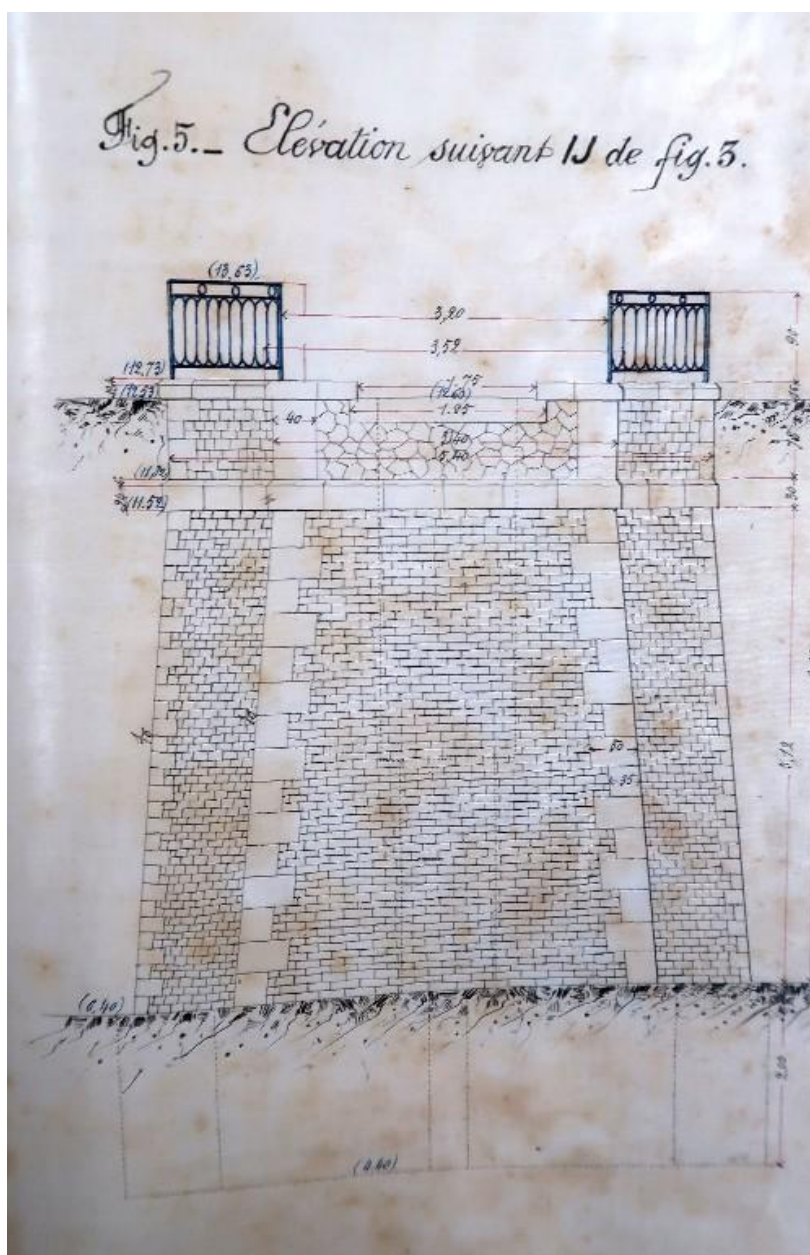
Elévation culée rive droite
