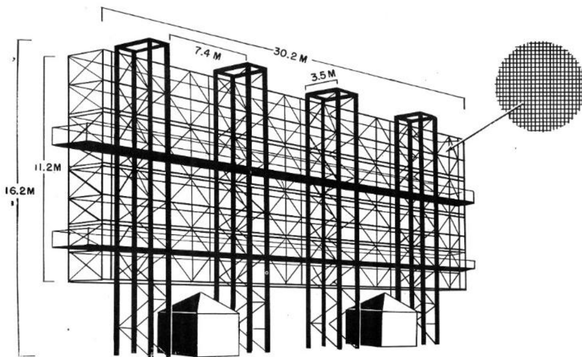
Dessin de l'antenne d'un radar Mammut (Hoarding radar, radar palissade) en version Lufwaffe à quatre mâts (extrait de War department technical manual, TM E11-219, Directory of German Radar Equipment, avril 1945)
