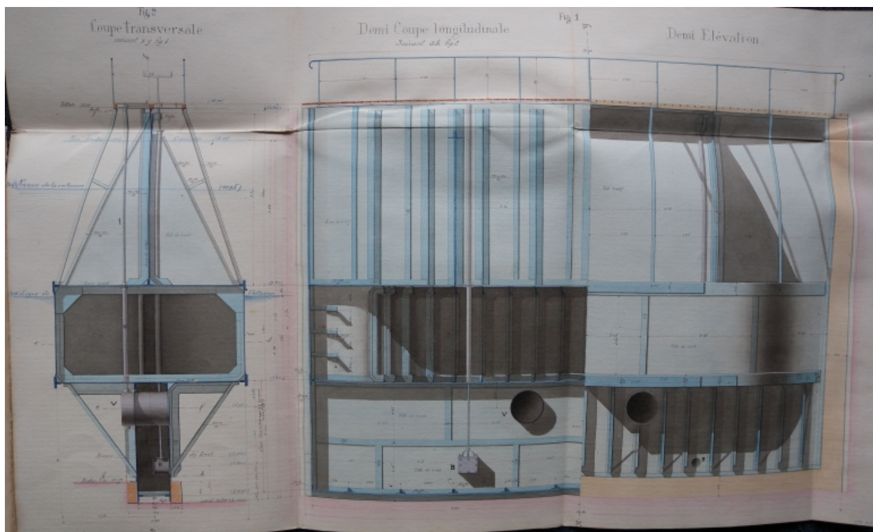
Plan : coupe transversale et longitudinale du bateau-porte, en projet, 1886 (AD 22)
