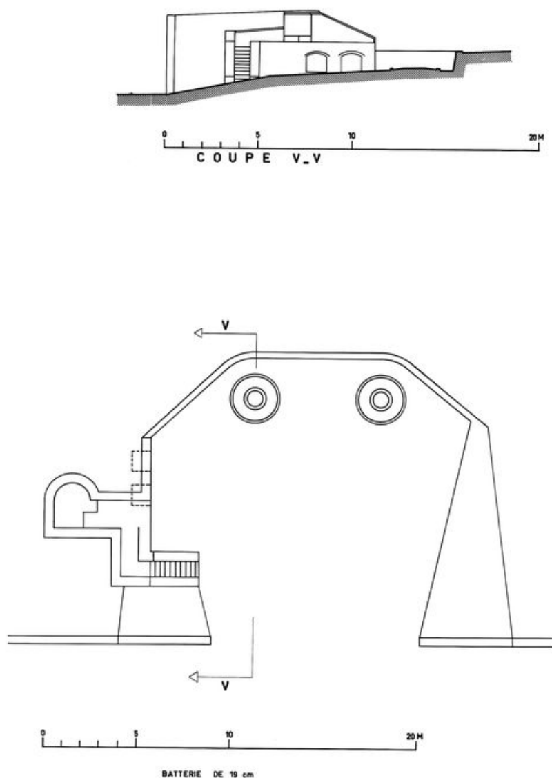
Coupe et plan de la batterie de 19 cm, le Toulinguet, Camaret-sur-Mer
