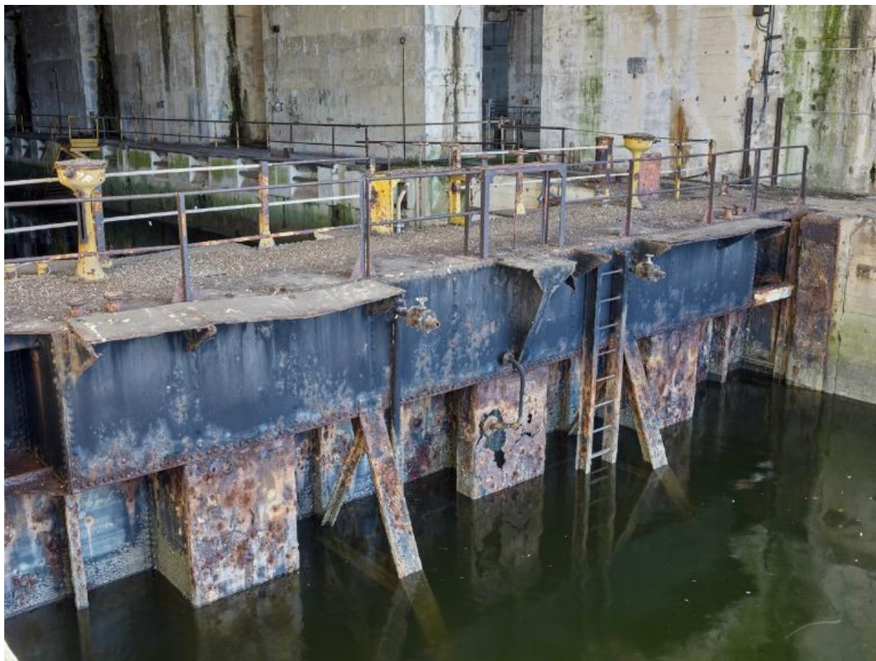
Vue du bateau-porte fermant le bassin depuis l'extérieur
