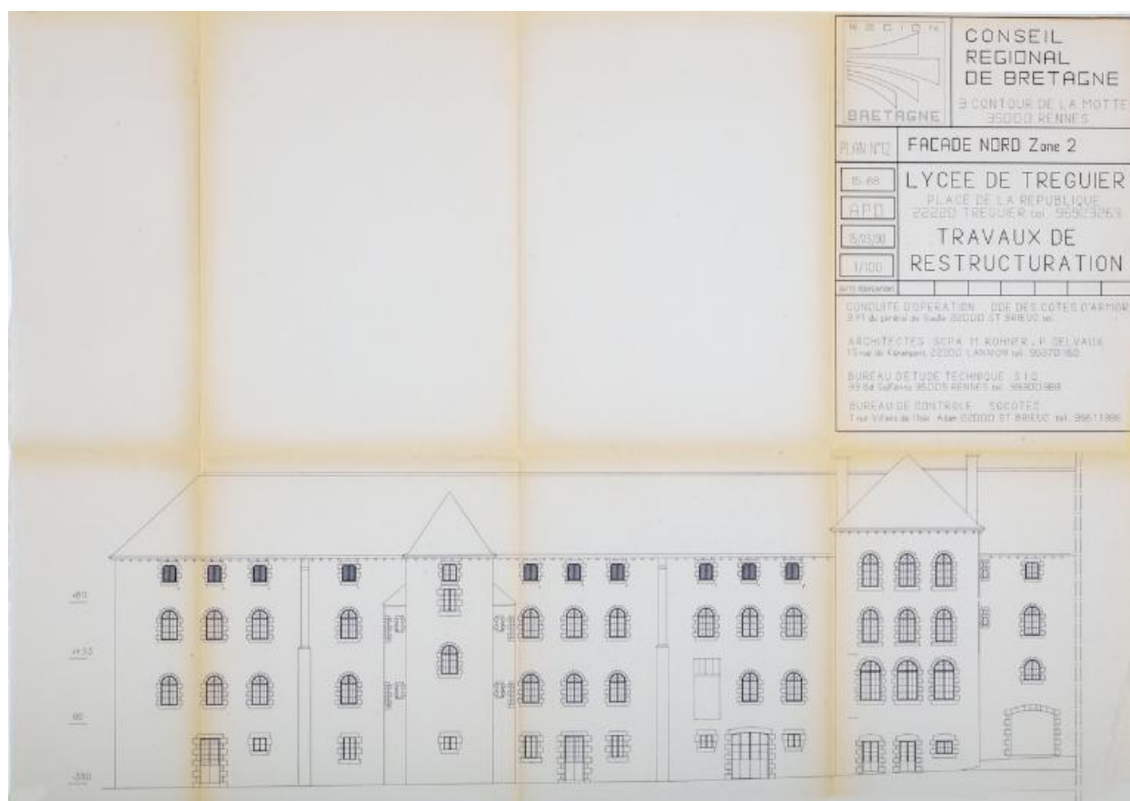
Tréguier : travaux de restructuration du lycée, zone 2, élévation nord (plan n° 12), 15 mars 1990 (Architectes SCPA : M. Rohner et P. Delvaux)
