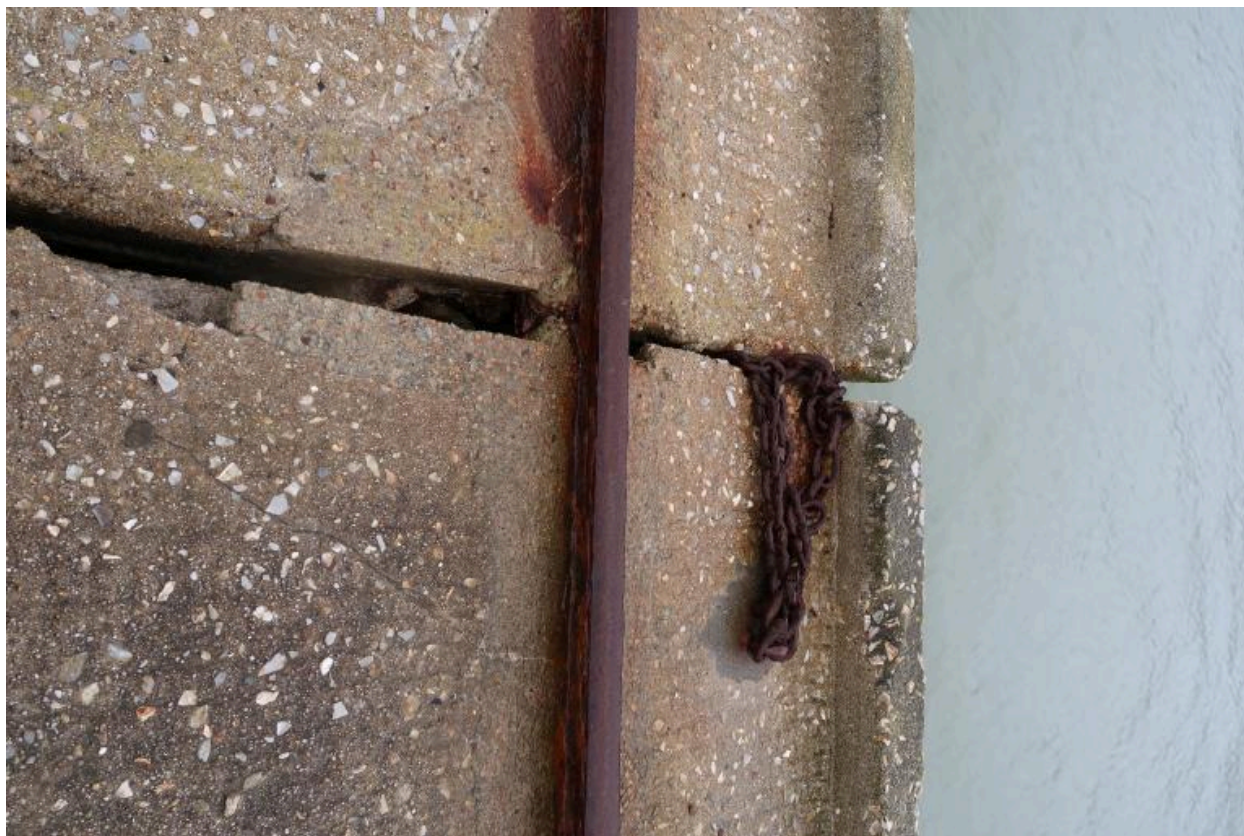
Rampe de lancement : jonction des dalles
