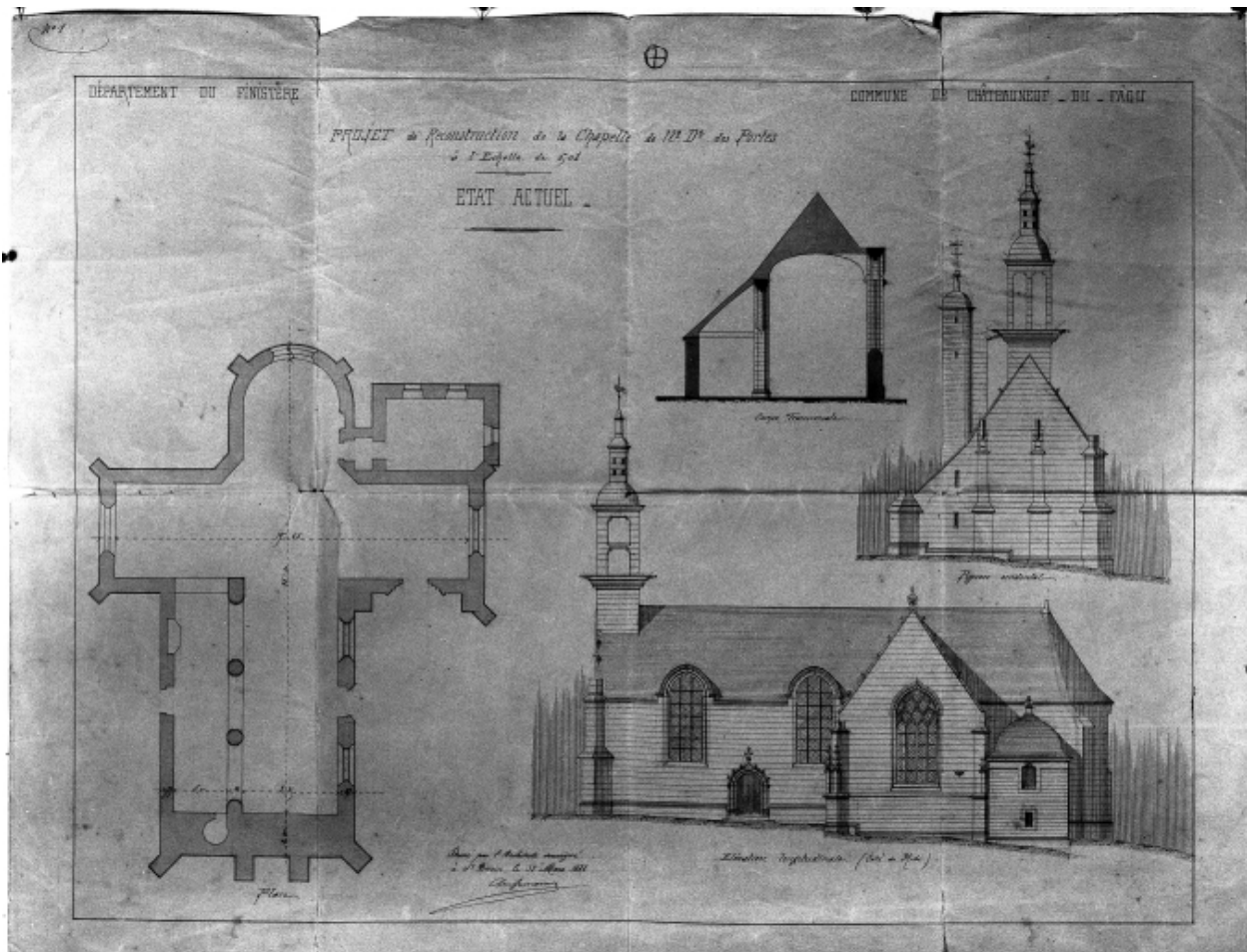
Châteauneuf-du-Faou, chapelle Notre-Dame-des-Portes : projet de reconstruction par Ernest Le Guerranic, 1888 (A.D. Finistère, 1 V 307)
