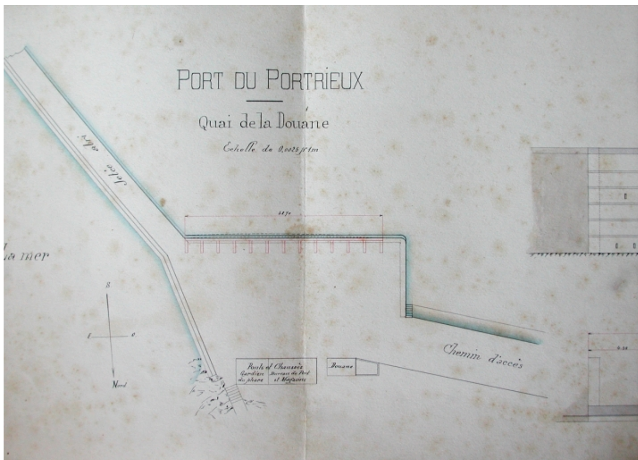
Plan, coupe et élévation : quai de la Douane, perpendiculaire à la jetée, 1911 (AD 22)
