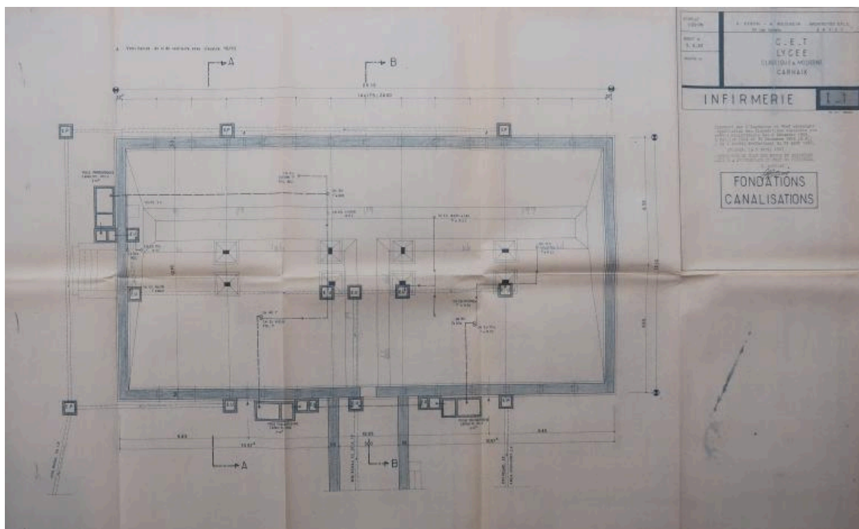
Plan des fondations et canalisations, H. Péron et A. Weisbein, architectes, 9/6/1965.
