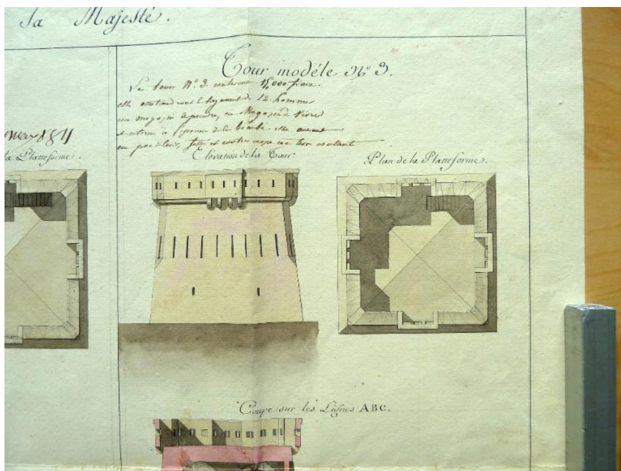
Plans, coupes et élévations des tours-modèles adoptées par sa majesté, 1811 : tour modèle n° 3 (pour 12 hommes)
