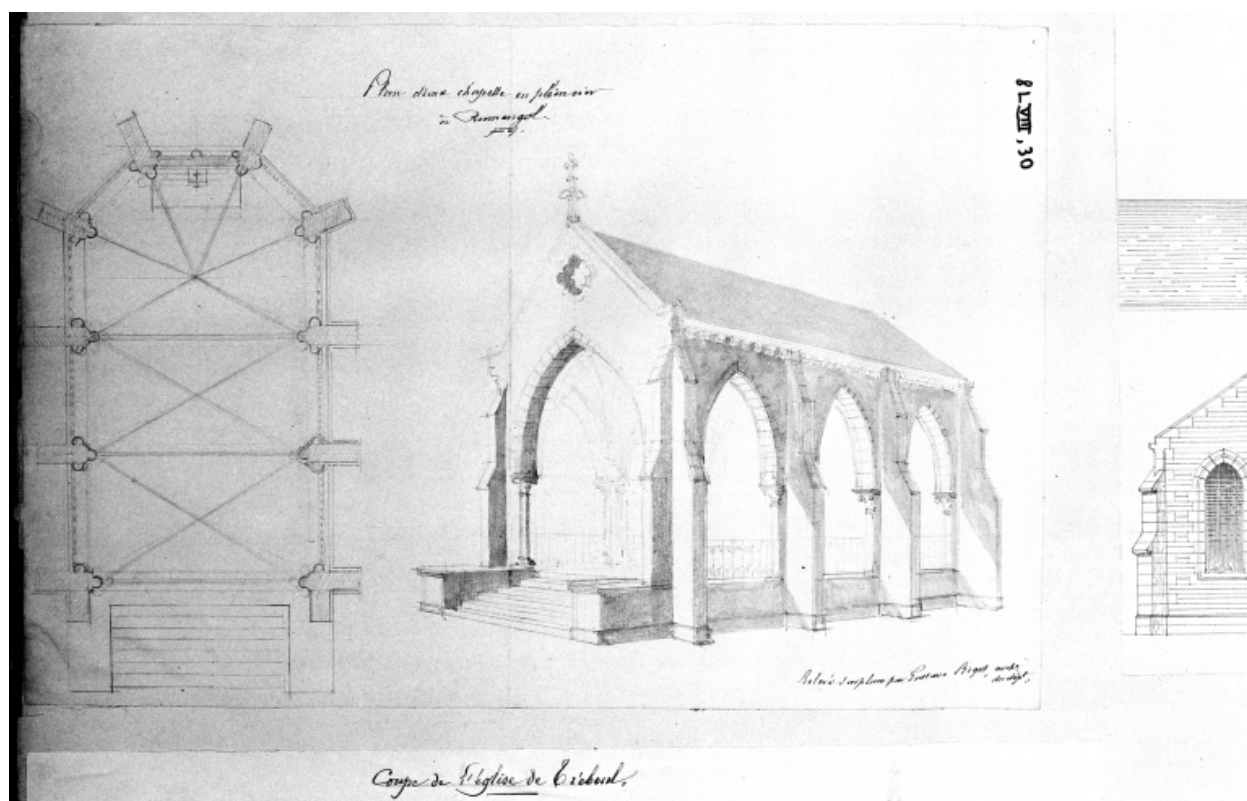
Plan et élévation de la chapelle de plein air. Projet de Gustave Bigot, 2e moitié 19e siècle (A. E. Quimper, 8 L XVIII 30)
