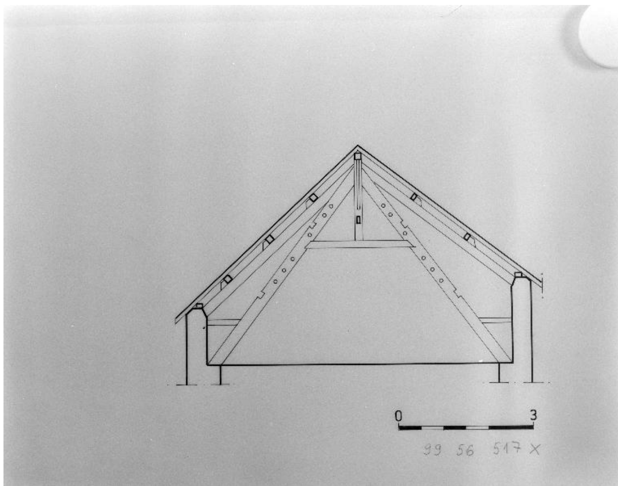
Coupe de la charpente.
