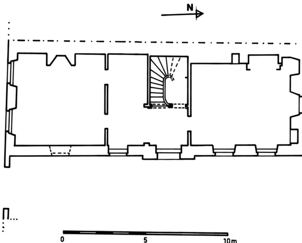
PLAN DU REZ - DE - CHAUSSEE
