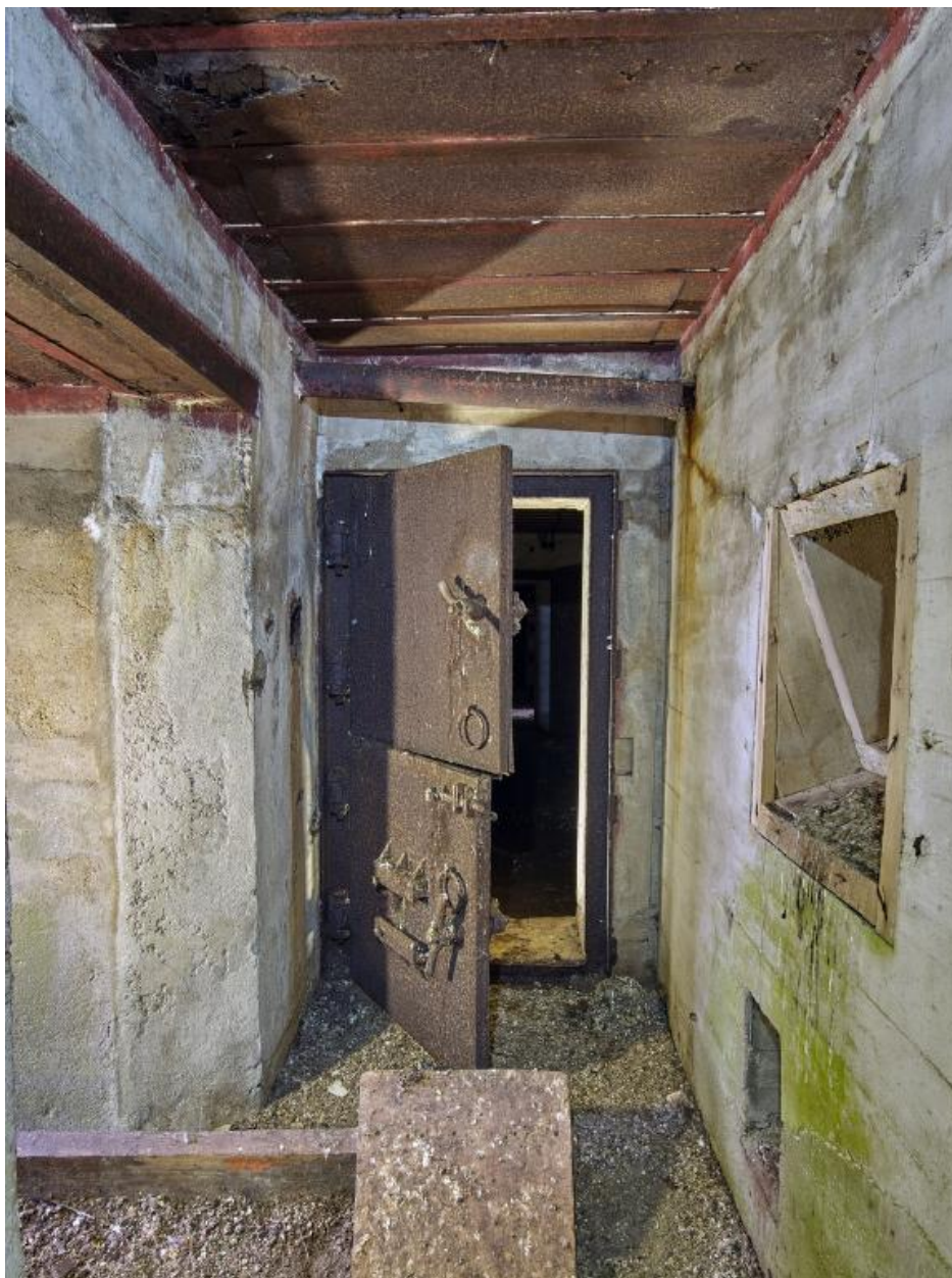
Vue intérieure : porte blindée à deux vantaux du sas. A gauche : couloir d'entrée ouest ; à droite : créneau de défense
