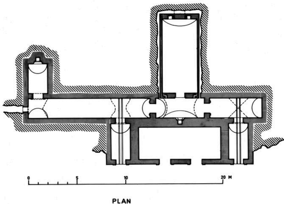
Plan du magasin sous roc de la batterie d'artillerie de la Droite des lignes de Quéléren
