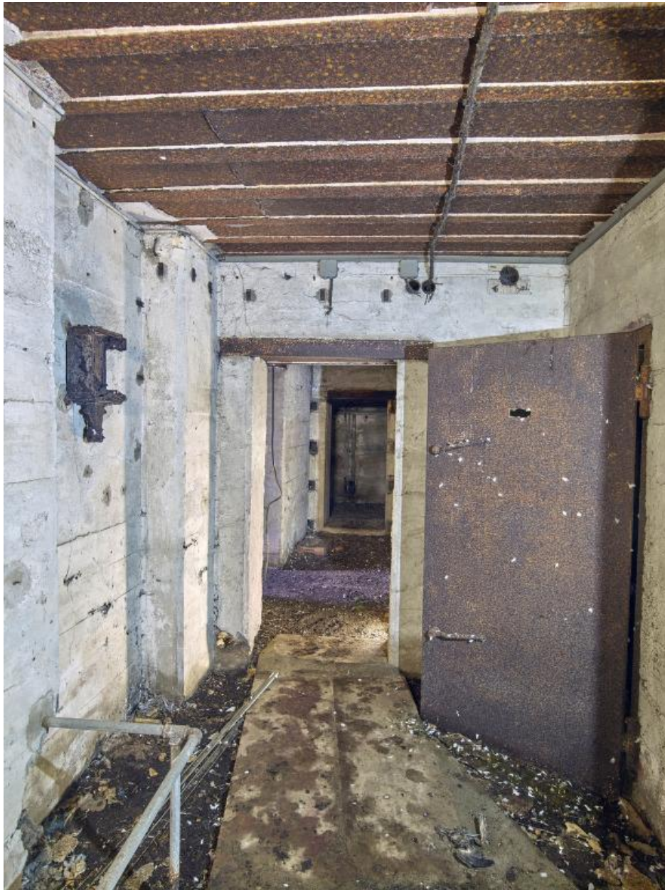
Vue intérieure : couloir du sas et porte étanche. Au fond du couloir, le magasin de munitions est
