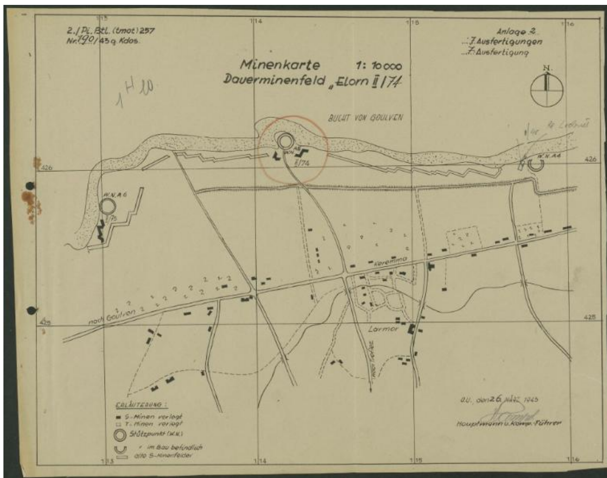
Dossier allemand de minage, commune de Tréfléz, champ de mines permanent Elorn II/74 : plan de situation, 26 mars 1943
