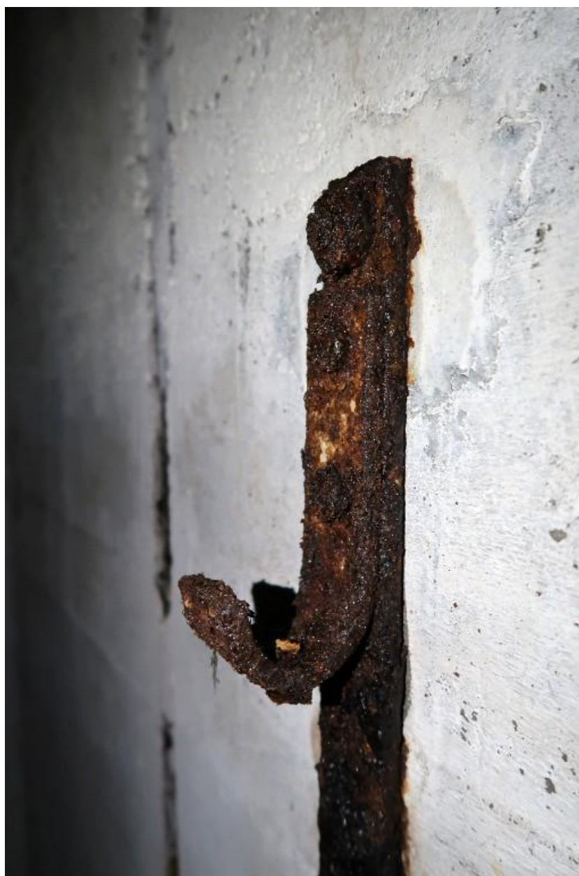
Vue de l'un des crochets muraux pour la fixation des couchettes tubulaires
