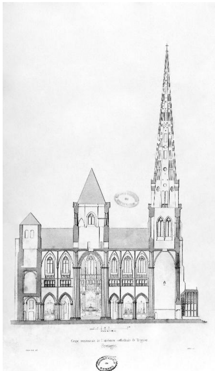
Tréguier : cathédrale Saint-Tugdual, coupe transversale
