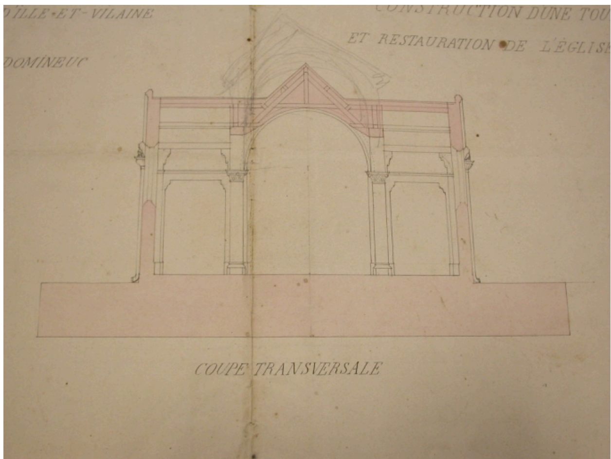
Coupe transversale
