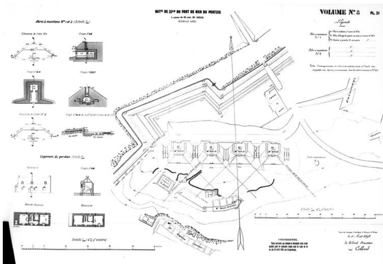
Plan et coupes de la batterie du fort de mer (4 canons de 32 cm), Direction d'Artillerie du génie de Brest, 1893, par le colonel Directeur d'Artillerie : Collomb
