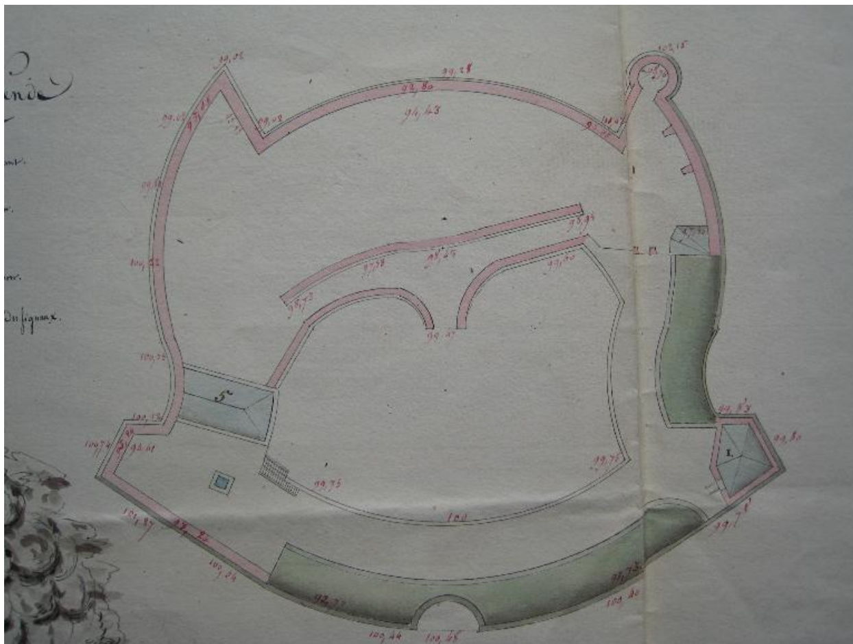
Plan du Fort Cigogne, daté du 20 octobre 1817 et signé Constantin, directeur des Fortifications, Colonel du Génie, Brest.
