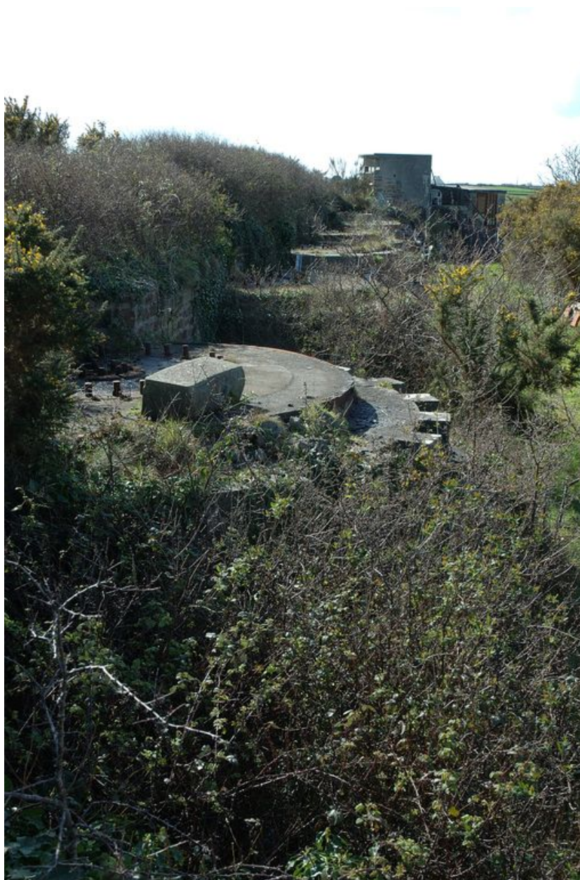
Vue de la batterie extérieure de 100 mm du Mengant : plate-formes pour pièce d'artillerie (état en 2007)
