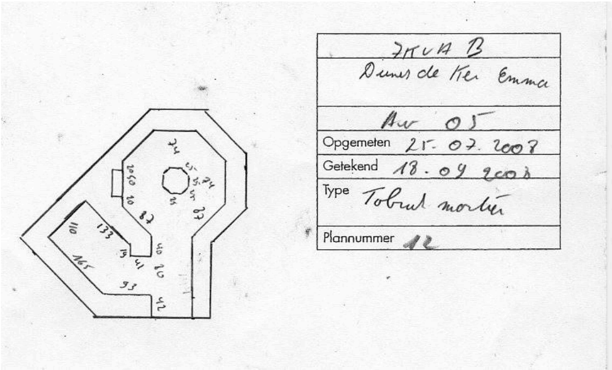
Plan du bunker-poste d'observation et de tir pour mortier dit Tobruk-Stand (dessin : Dirk Peeters)
