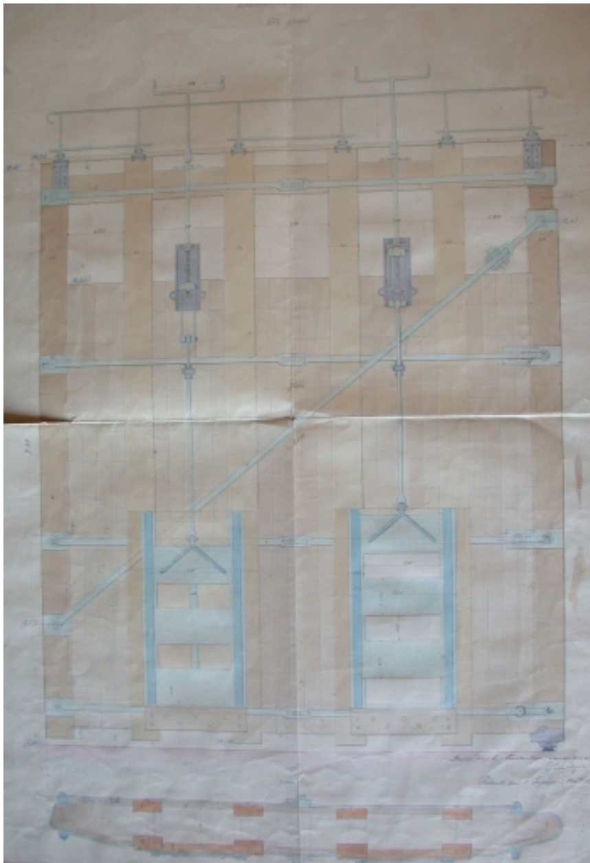
Dessin : élévation d'un vantaux de la 1ère écluse, face amont, 1875 (AD 22)
