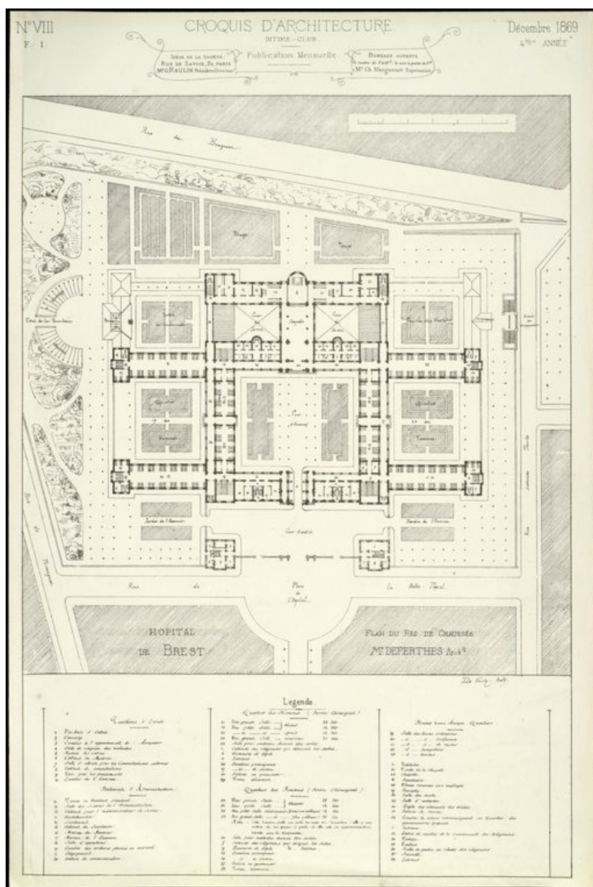
Projet d'hôpital pour Brest par Edouard Deperthes, architecte de la ville de Brest : plan général et légende, Intime-club, croquis d'architecture, publication mensuelle, décembre 1869
