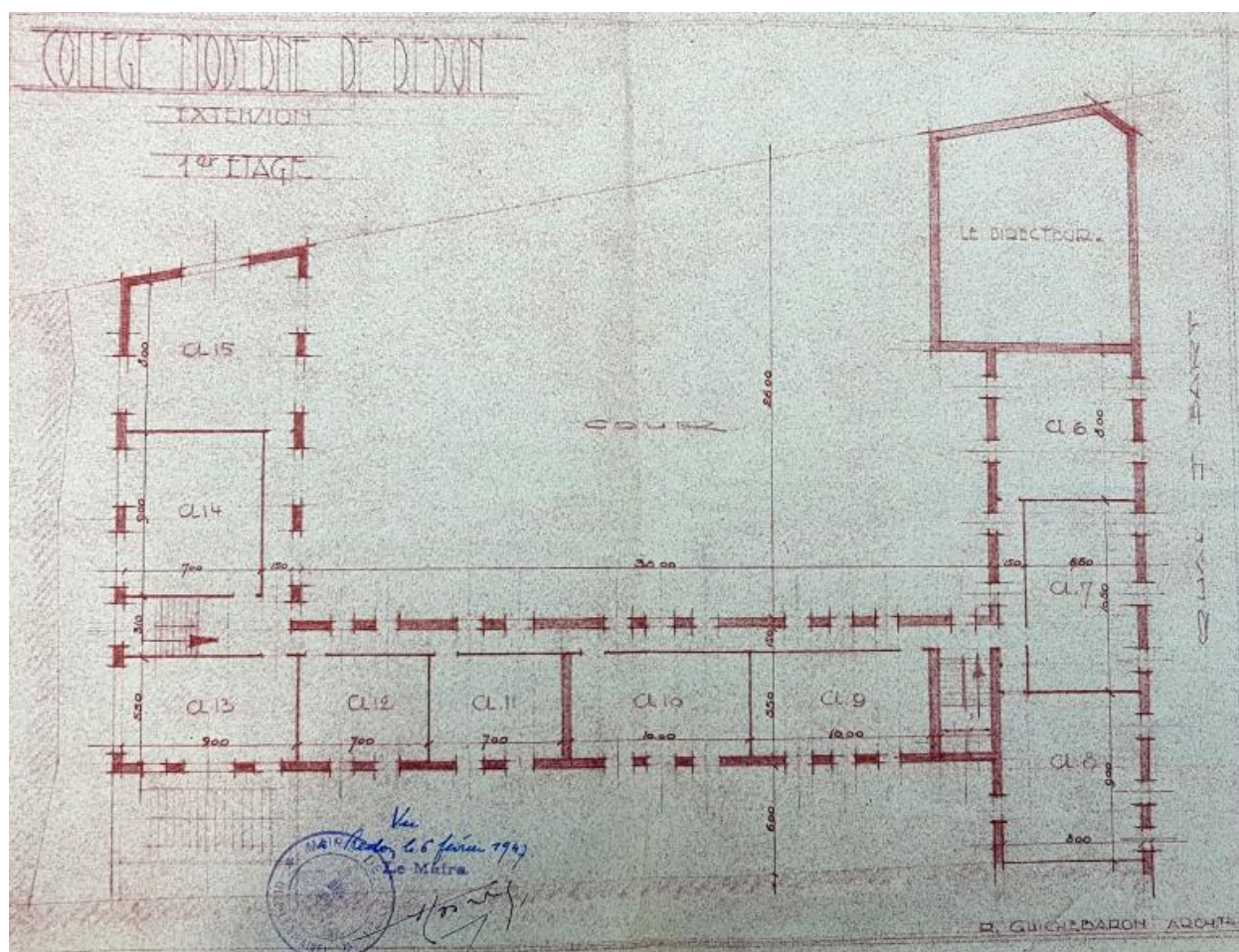
Collège moderne de Redon. Extension. 1er étage. R. Guichebaron, architecte, 1947
