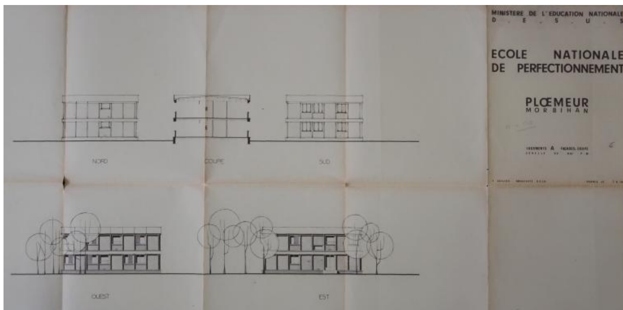
Logements A, façades - coupe. Yves Guillou, architecte, 1967.
