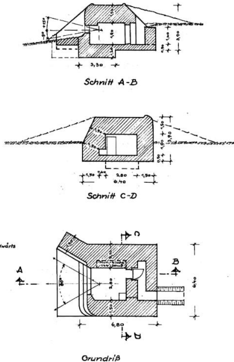
Plan-type d'un bunker de type 667 (Kleinstschartenstand für 5cm KwK)
